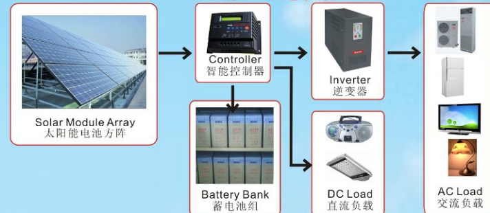
太阳能独立发电系统图
