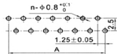
反针 PCB 寸法 Versa needle PCB LAYOUT
