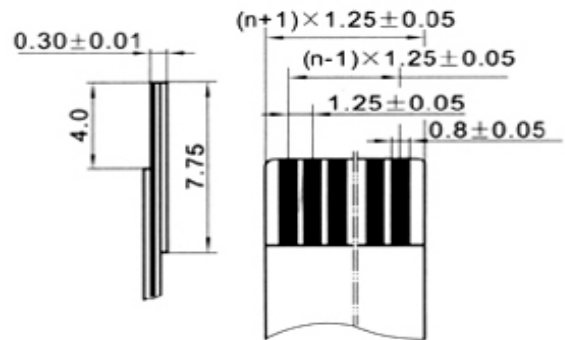
适用扁平电缆 Proper cable
