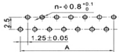
正针 PCB 寸法 Positive needle PCB LAYOUT
