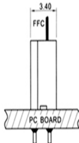
安装图 ASSEMBLY LAYOUT
