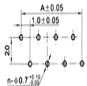
反针 PCB 寸法 Versa needle PCB LAYOUT
