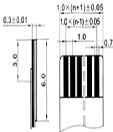
适用扁平电缆 Proper cable
