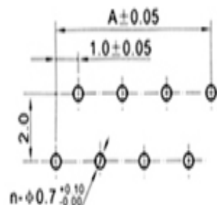
正针 PCB 寸法 Positive needle PCB LAYOUT
