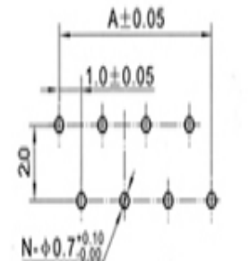
反针 PCB 寸法 Versa needle PCB LAYOUT
