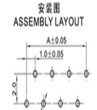
正针 PCB 寸法 Positive needle PCB LAYOUT
