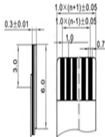
适用扁平电缆 Proper cable
