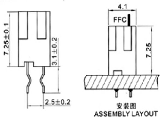
适用扁平电缆 Proper cable
