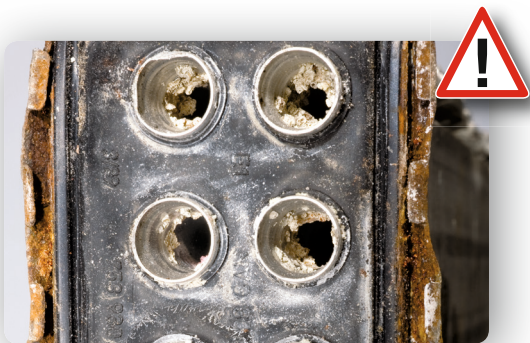
散热器中的水垢
