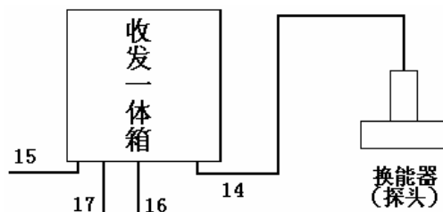
图 9 电缆配置图
