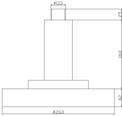
常温型换能器
