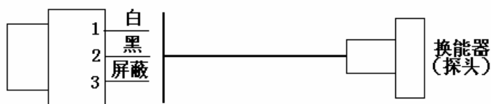
图 10 14 号电缆图
