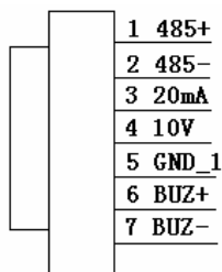
图 12 16 号电缆配置图
