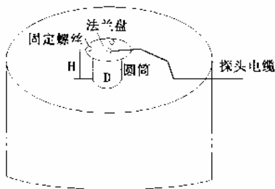
图3 密封仓安装示意图
