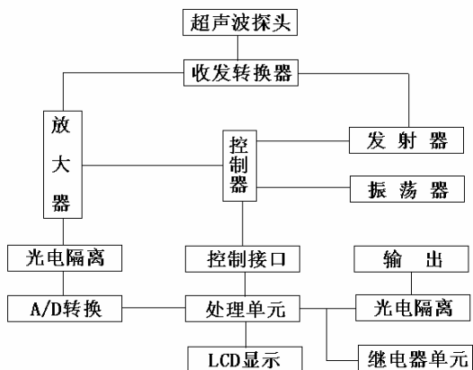
图 1、系统框图
