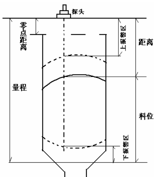
图 16 参数示意图
