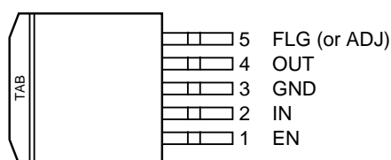
LM39301-x.x, LM39302BU TO-263-5 (U)
