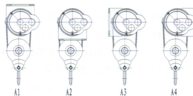
CD/MD, 型固定式 Model CD 1 /MD 1 Stationary
