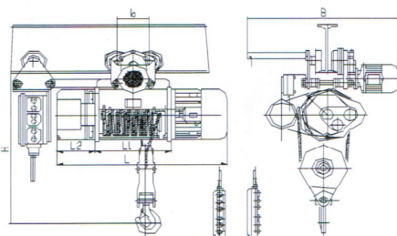
HB型 0.25-5吨(H=6-9米) Model HB 0.25-5T(H=6-9m)
