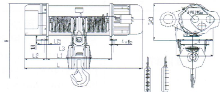
HB型 固定式 10吨(H=9-30米) Model HB Stationary 10T (H=9-30m)
