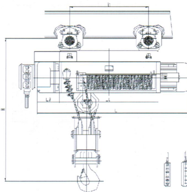
HB型 16吨(H=9-30米) Model HB 16T(H=9-30m)
