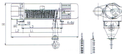
HB型 固定式 0.5-5吨(H=12-30米) Model HB Stationary 0.5-5T(H=12-30m)
