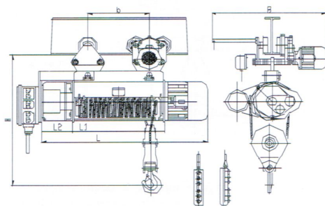
HB型 0.5-5吨(H=12-30米) Model HB 0.5-5T(H=12-30m)
