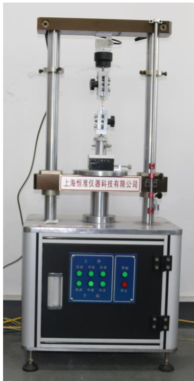
Servo Tensile Testing Machine
