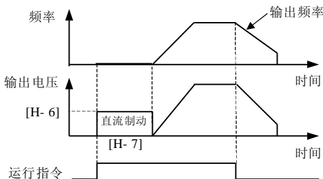
图 8-17 启动直流制动功能
