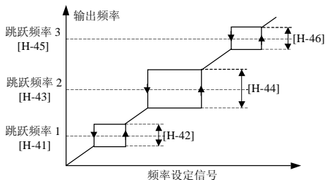
图 8-22 跳跃频率及幅度示意图
