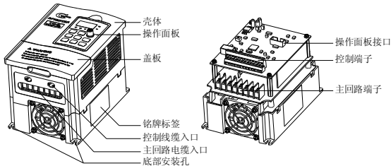
图 2-2 变频器部件名称
