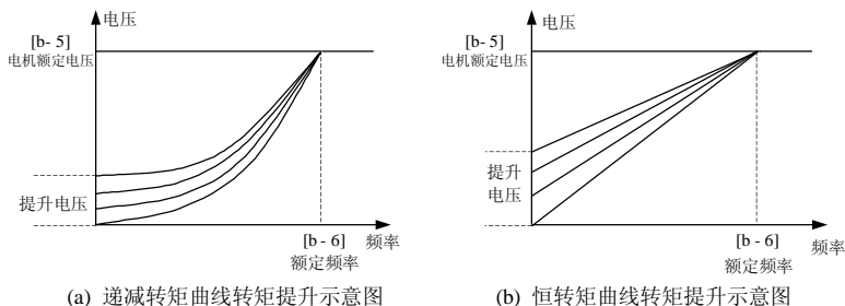
图 8-7 转矩提升示意图
