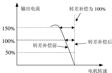
图 8-15 转差频率补偿示意图
