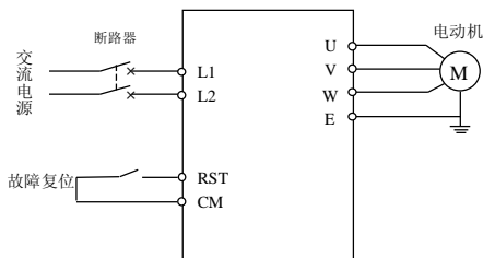
图 6-1 简单运行接线图
