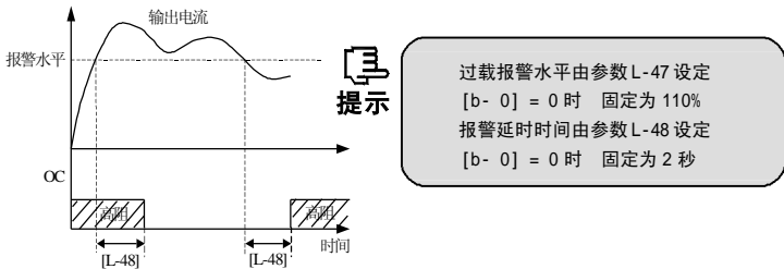
图 8-5 过载报警
