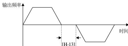
图 8-19 正反转死区时间
