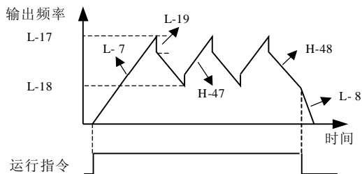
8-20 摆频运行
