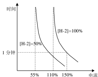
图 8-16 电子热继电器保护
