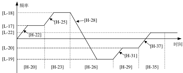
图 8-21 可编程多段速运行
