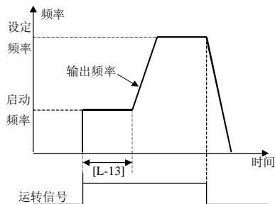
图 8-11 启动频率运行
