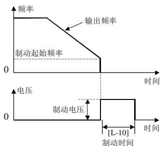
图 8-10 直流制动功能
