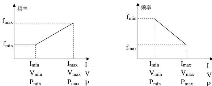
图 8-14 输入量与设定频率的对应关系
