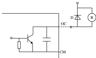
图 8-2 OC 的内部接线图
