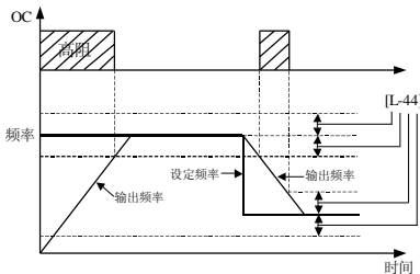
图 8-3 频率到达信号
