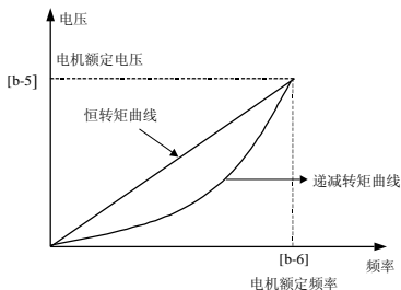
图 8-6 V/F 曲线
