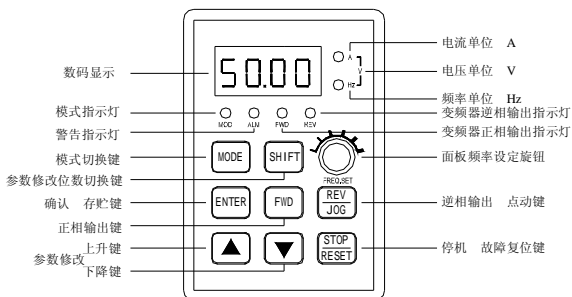
图 5-1 操作面板布局图
