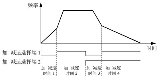
图 8-23 加 减速时间选择
