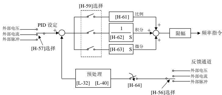
图 8-24 内藏 PID 控制
