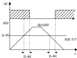
图 8-4 频率水平检测(FDT)
