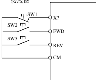
图 8-18 三线控制模式接线图
