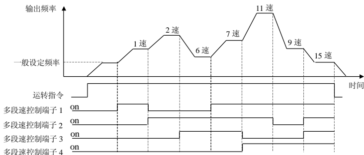
图 8-13 多段速运行示意图
