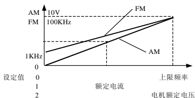
图 8-1 AM FM 端子的表示内容
