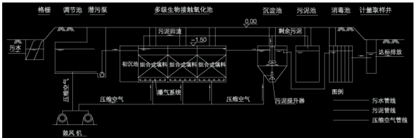
地理式生活污水处理成套设备工艺流程图
