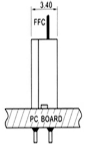
安装图 ASSEMBLY LAYOUT
