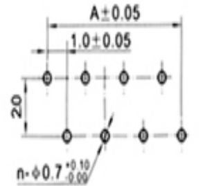
反针 PCB 寸法 Versa needle PCB LAYOUT
