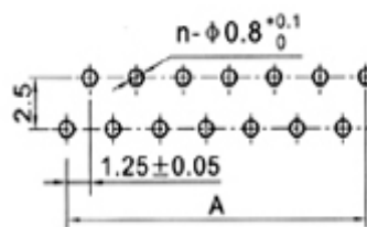
正针 PCB 寸法 Positive needle PCB LAYOUT
