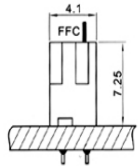
安装图 ASSEMBLY LAYOUT
