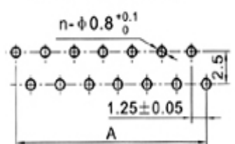
反针 PCB 寸法 Versa needle PCB LAYOUT
