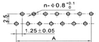
正针 PCB 寸法 Positive needle PCB LAYOUT
