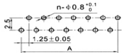
正针 PCB 寸法 Positive needle PCB LAYOUT
