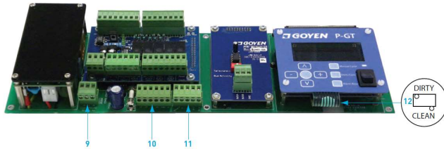
PGT-ACDC 主控制器模块
