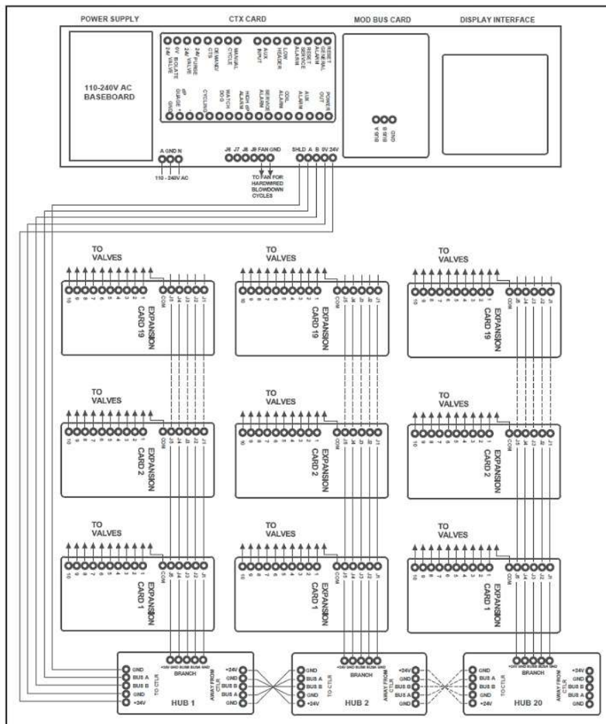
主板与付板的接线
