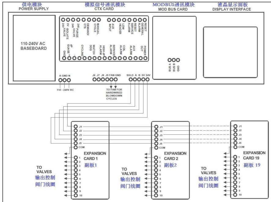
主板与付板的接线
