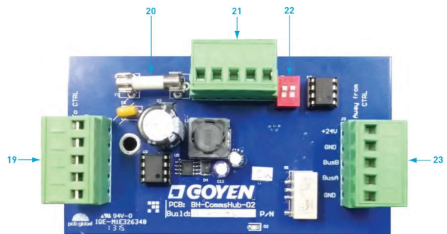
HUB 付板地址分配模块
