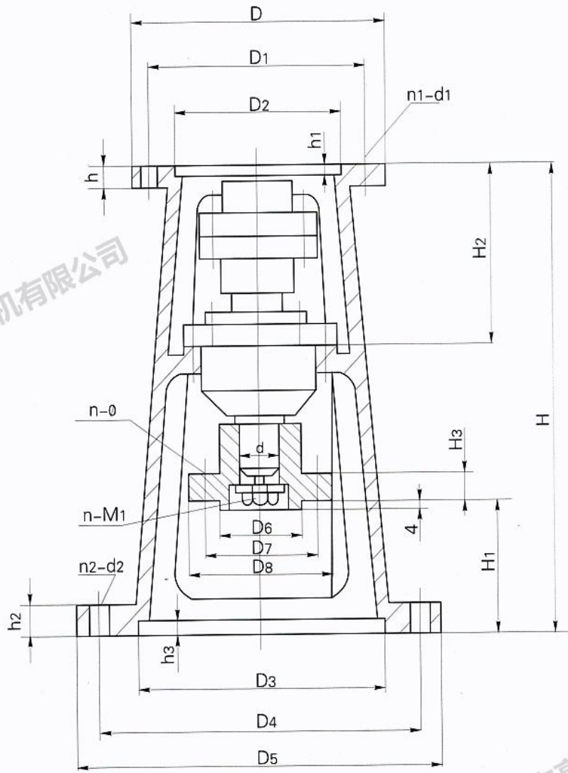
图5-5 TJ型机架
