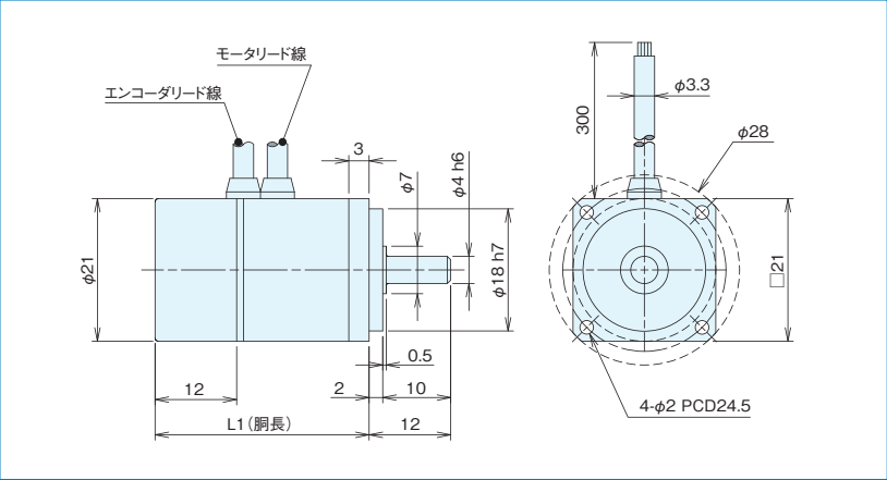
外形寸法図
