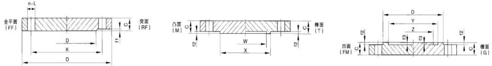
钢制管法兰（盲板）BL（HG20601-97、JB/T86-94、GB/T9123-2000）
