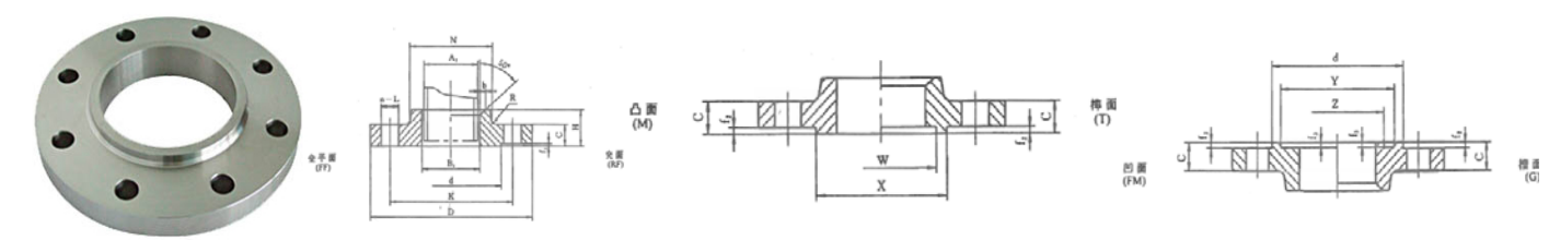
带颈平焊钢制管法兰（HG20594-97、GB/T9116-2000）
