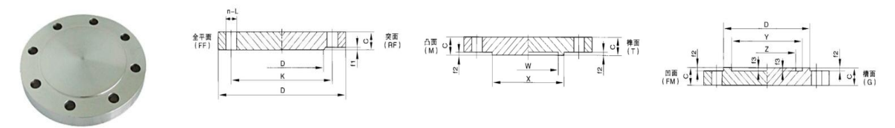
钢制管法兰（盲板）BL（HG20601-97、JB/T86-94、GB/T9123-2000）
