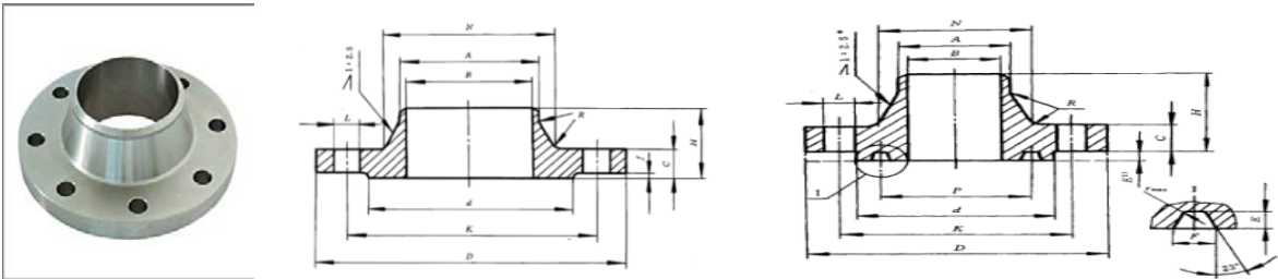
带颈对焊钢制管法兰（HG20595-97、JB/T82.1-94、GB/T9115.1-2000）
