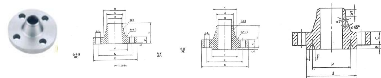
美标带颈对焊钢制管法兰WN（ASME B16.5、HG 20616-97）
