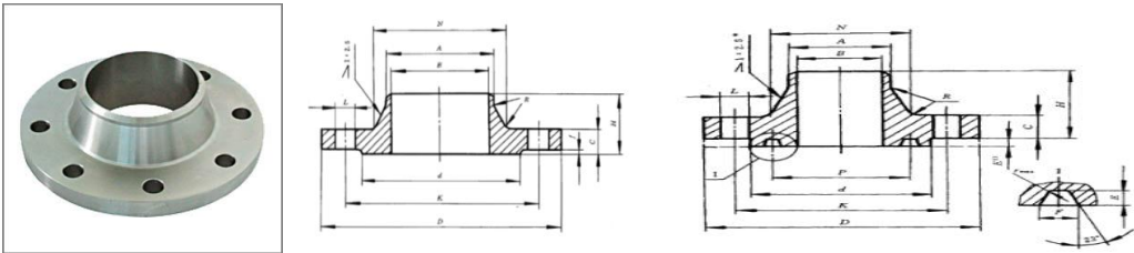
带颈对焊钢制管法兰（HG20595-97、JB/T82.1-94、GB/T9115.1-2000）
