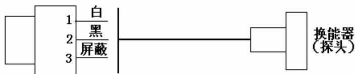
图 10 14 号电缆图
