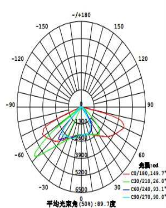
子午面配光曲线
