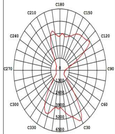
最大光强处圆锥面光强分布曲线
