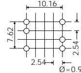
印刷電路板佈局 (頂視圖)
