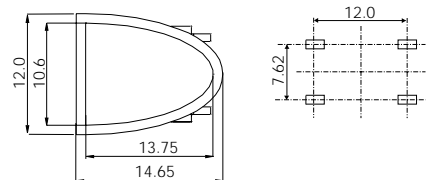
印刷電路板佈局
